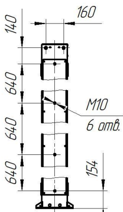
Места для крепления к турникету полноростовых ограждений «Ростов-Дон» (вид на стойки 1 и 2 справа и слева)
