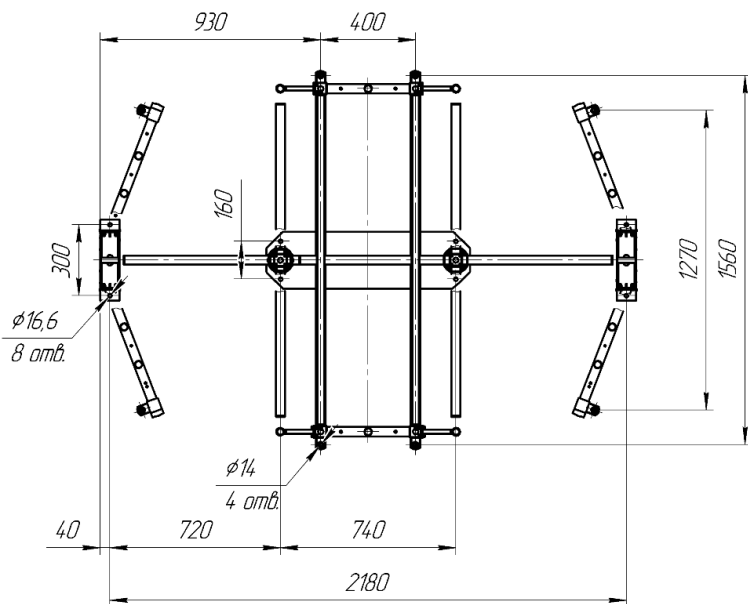
Установочные размеры турникета «Ростов-Дон PR2/4M2»
